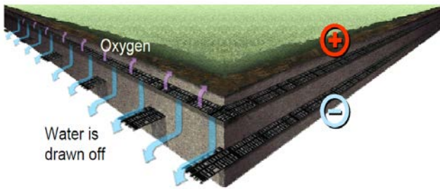
圖十一 EKG 草皮配置圖(Jones 等人，2008)
