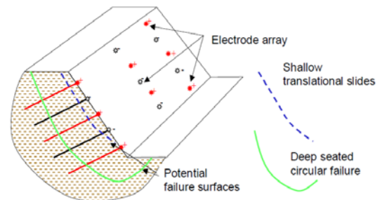
圖七 電滲透原理強化坡面穩定性示意圖(Jones 等人, 2008)
