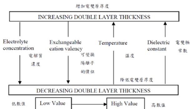
圖三 影響電雙層厚度因素(Pugh, 2002)
