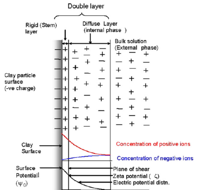
圖二 電雙層示意圖(Jones 等人, 2008)
