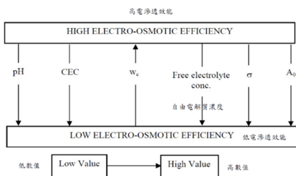
圖四 影響電滲透效能之土壤參數(Jones 等人, 2008)
