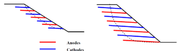
圖八 電滲透 EKG 土釘淺層(左圖)與深層穩定工法陰陽極配置示意圖(Jones 等人, 2008)
