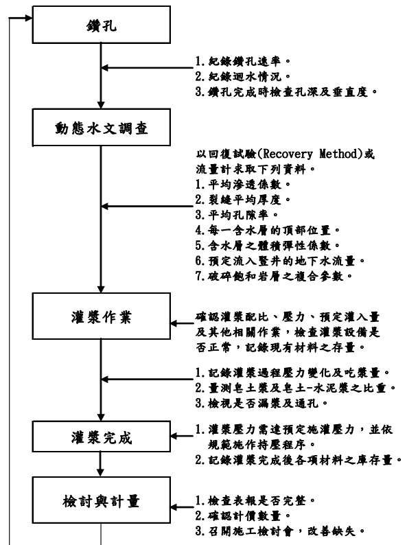
圖二 豎井工程灌漿程序流程圖
