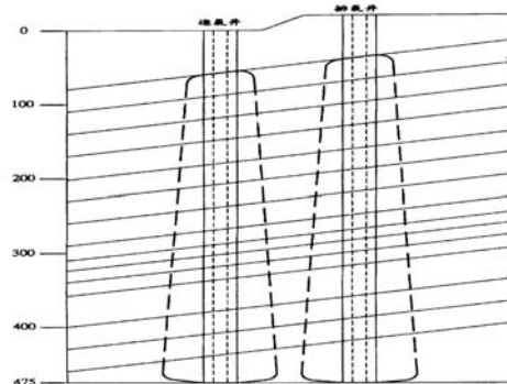
圖四 一號豎井皂土水泥灌漿帷幕剖面示意圖
