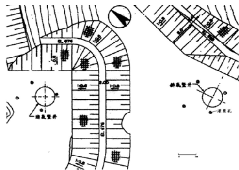
圖三 一號豎井皂土水泥灌漿佈孔圖
