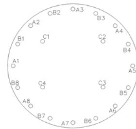
圖五 三號豎井 L.W 灌漿孔配置圖
