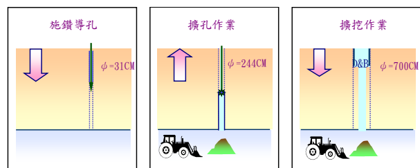
圖七 昇井工法施工步驟圖
