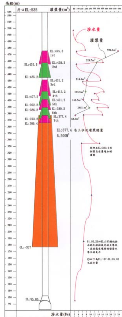
圖九 三號豎井進氣井 L.W.灌漿量與滲水量關係圖
