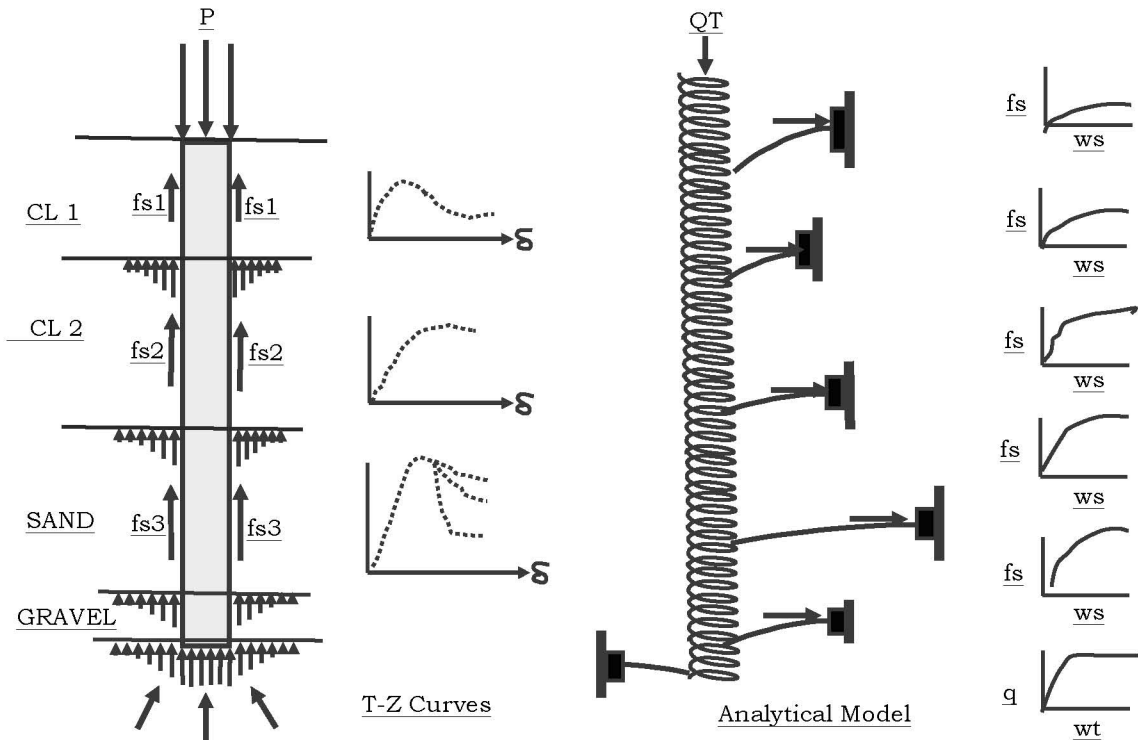
圖十 使用 T-Z 曲線分析基樁荷重-位移行為模式
